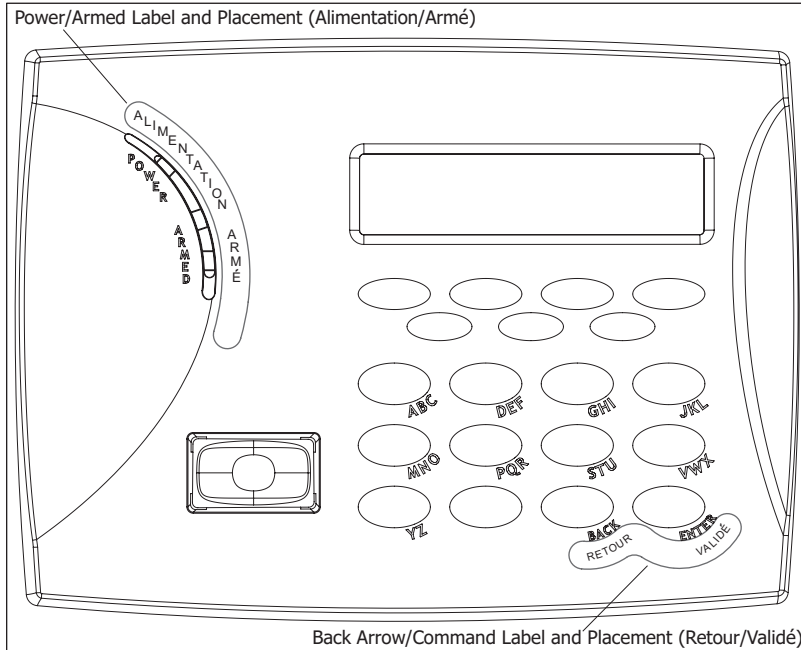
Figure 1: Thinline Keypad with French Text Labels Installed Figure 1: Clavier Thinline avec étiquettes françaises.
